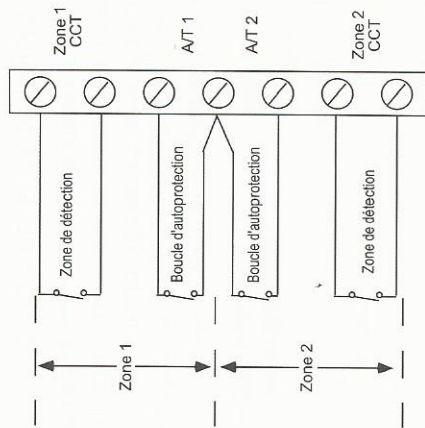
Figure 9. Raccordement 4 fils des détecteurs (détection/autoprotection)
